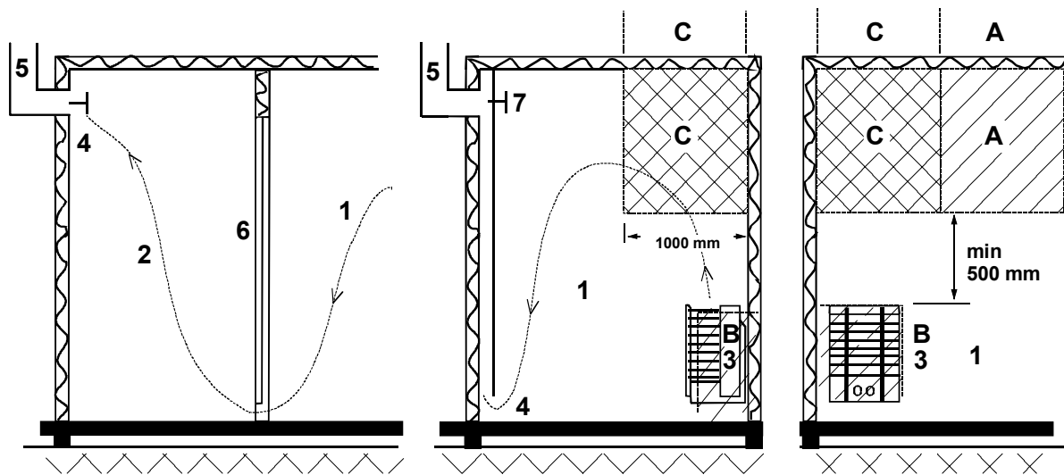
Рисунок 1. Вентиляция сауны
