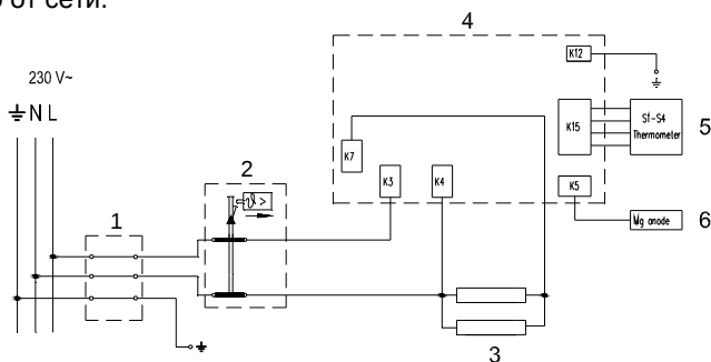
Электросхема
