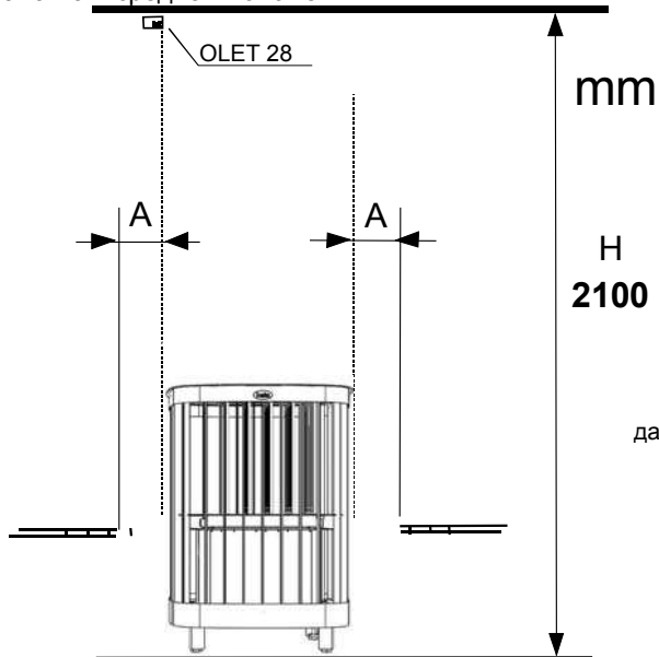
Рис. 7 Установка в среднем положении
