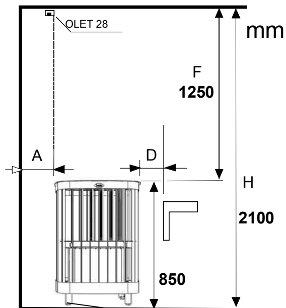
Рис. 6 Угловая и настенная установка
