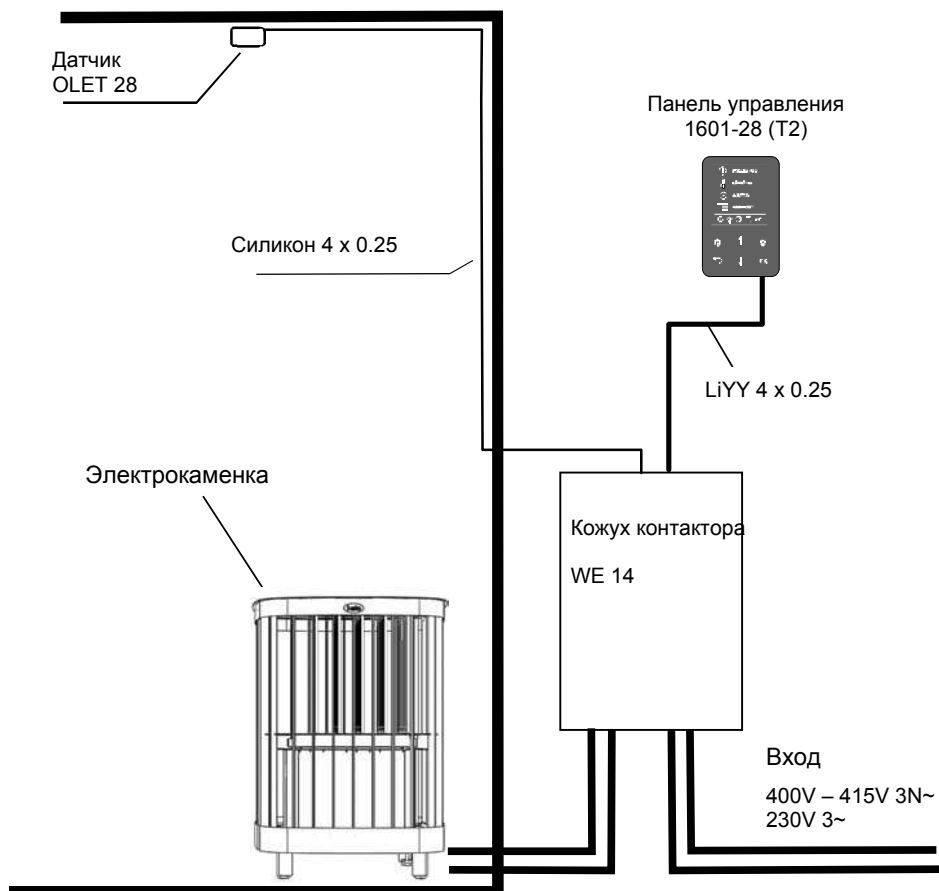
Рис. 8 Принципиальная схема соединений
