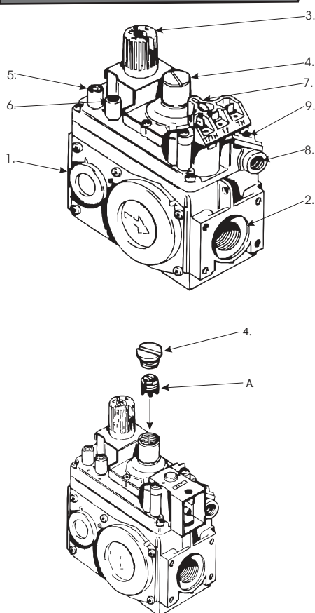
Комбинированная газовая арматура SIT - NOVA
