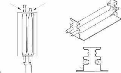
Рис 10 | Расположение датчика Fig. 10 | Sensor Location
