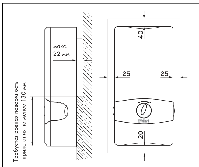
Рис. 5.1 Свободные пространства
