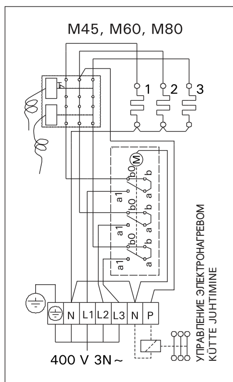
Рисунок 12. Электромонтаж каменки М Joonis 12. M-kerise elektriühendused
