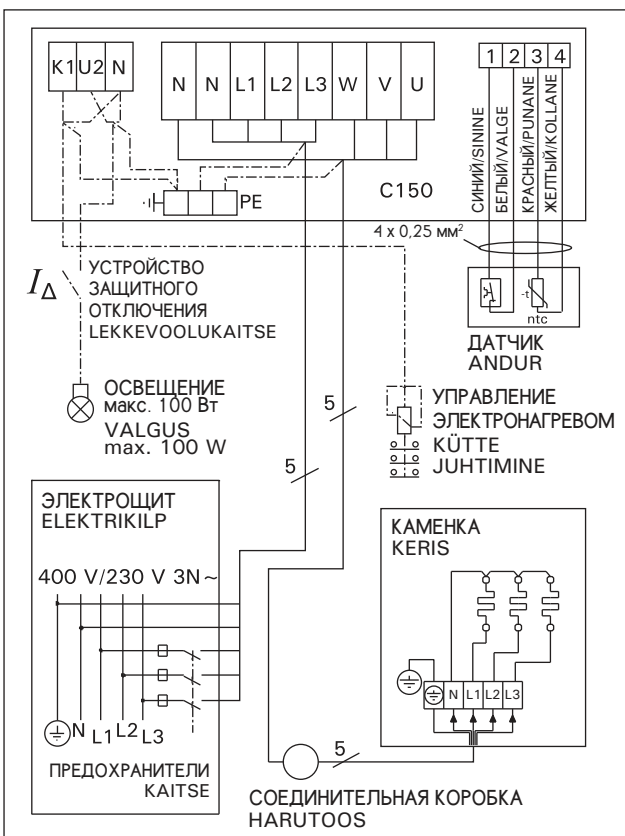
Рисунок 18. Электромонтаж пульта управления C150 и каменки M-E (подключение в 3- фазной сети) Joonis 18. Juhtimiskeskuse C150 ja M-E-kerise 3- faasilised elektriühendused
