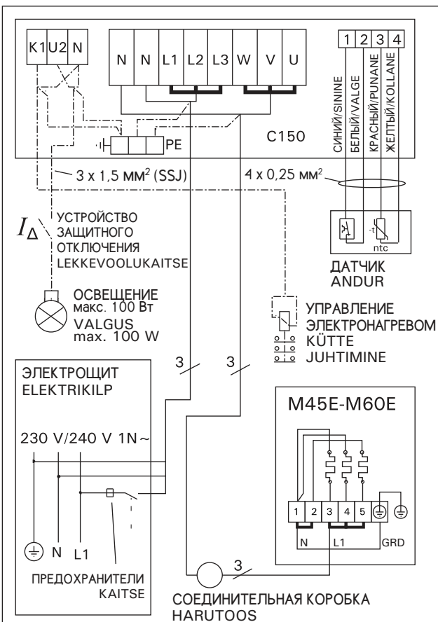
Рисунок 16. Электромонтаж пульта управления C150 и каменки M-E (подключение в 1-фазной сети) Joonis 16. Juhtimiskeskuse C150 ja M-E-kerise 1-faasilised elektriühendused
