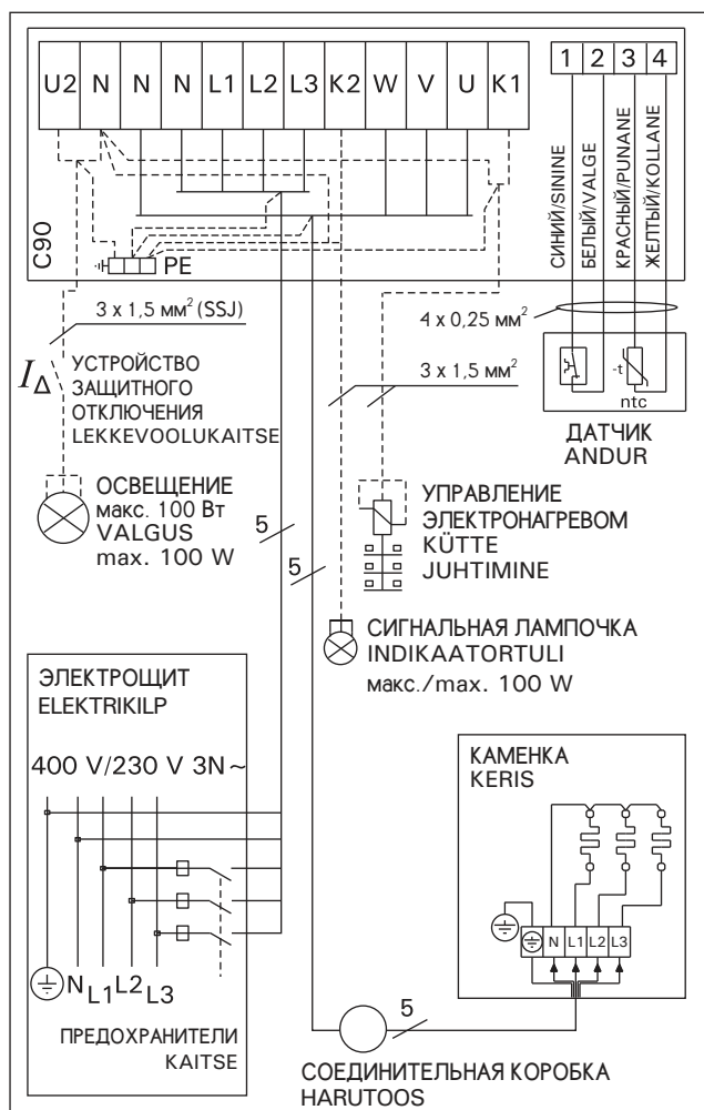
Рисунок 17. Электромонтаж пульта управления C90 и каменки M-E (подключение в 3- фазной сети) Joonis 17. Juhtimiskeskuse C90 ja M-E-kerise 3- faasilised elektriühendused
