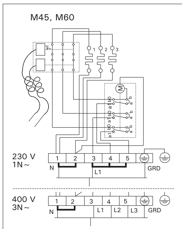
Рисунок 13. Электромонтаж каменки М Joonis 13. M-kerise elektriühendused
