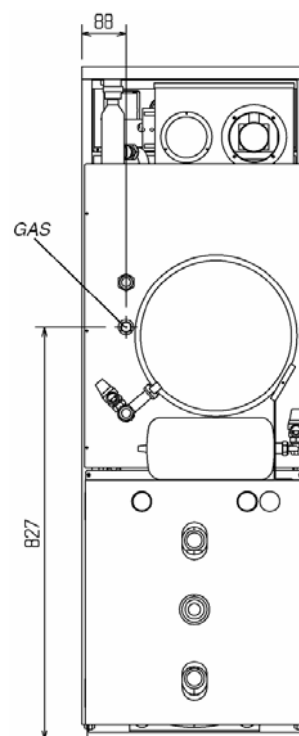
Fabula 32 csi 80
