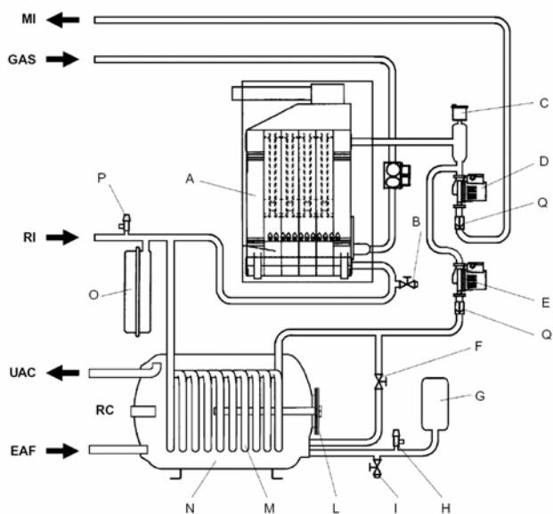
Fabula 32 csi 80
