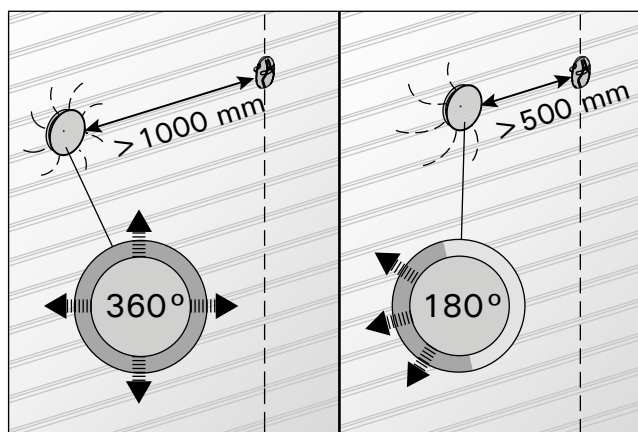
Рисунок 6. Минимальное расстояние между датчиком и вентилятором Joonis 6. Anduri minimaalne kaugus ventilatsioonist
