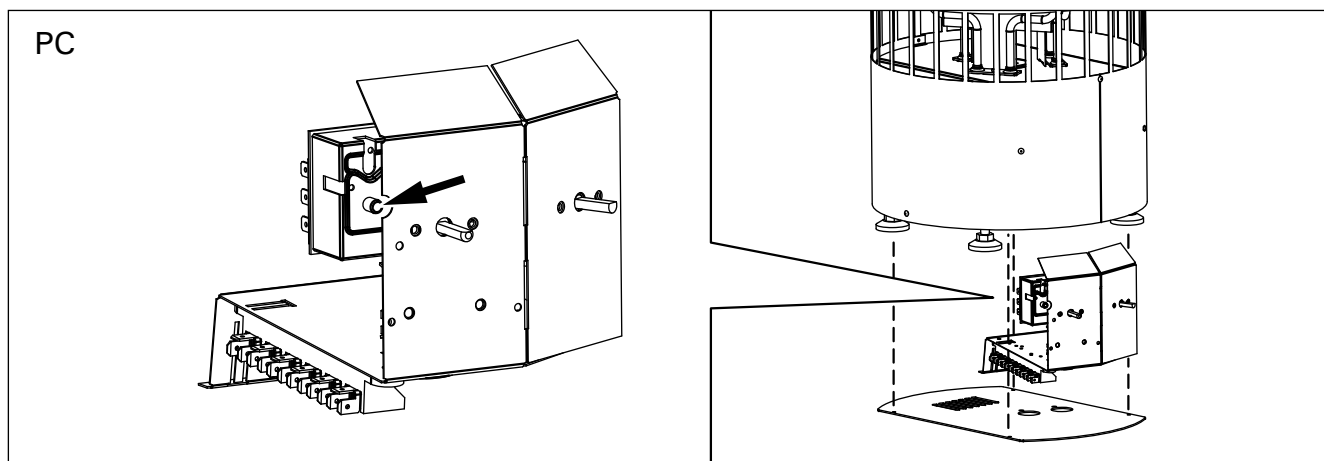
Рисунок 9. Кнопка сброса защиты от перегрева
