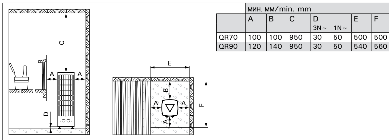
Рисунок 6. Расположение и безопасные расстояния (все размеры приведены в миллиметрах)
