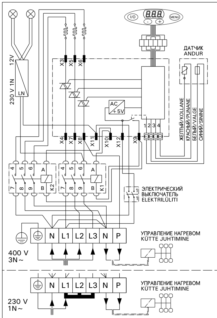
Рисунок 10. Подключение каменок FU Joonis 10. Keriste FU elektrüühendused
