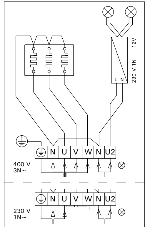
Рисунок 11. Подключение каменок FU-E Joonis 11. Keriste FU-E elektrüühendused
