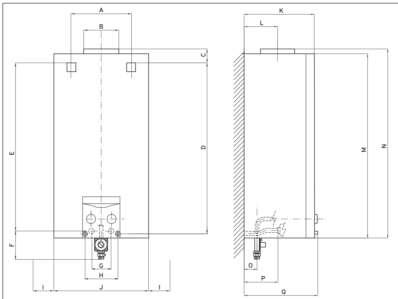
Рис. 4.3 Размеры водонагревателя атмоMAG 14-0/0 RXZ для природного газа
