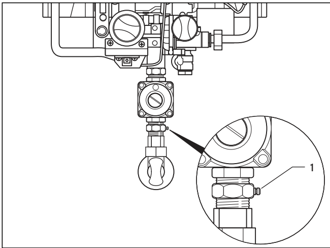
Мал. 6.1 Вимірний штуцер приєднувального тиску газу
