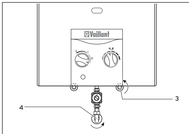
Рис. 4.2 Запорные устройства
