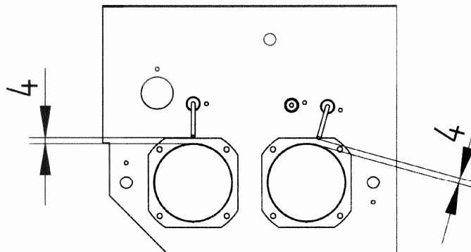
Рис. 26 Розташування електродів запалення
