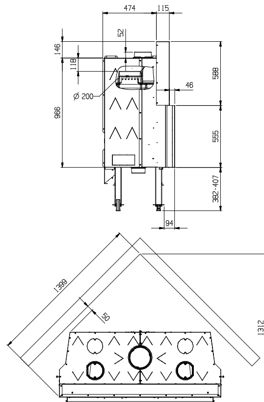
1300 - MONOBLOCCO PIANO
