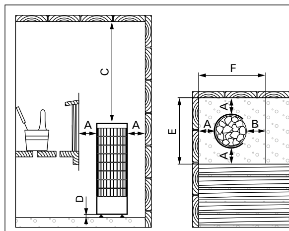
Рисунок 4. Расположение и безопасные расстояния (все размеры приведены в миллиметрах) Joonis 4. Ohutuskauused (kõik mõõtmised millimeetrites)
