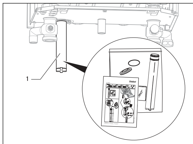
Рис. 5.12 Заполнение сифона
