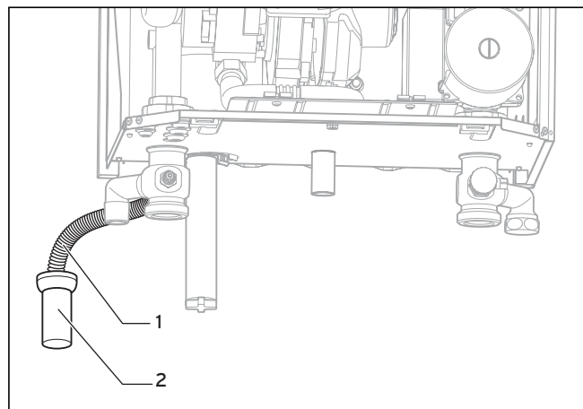
Рис. 5.11 Отвод конденсата
