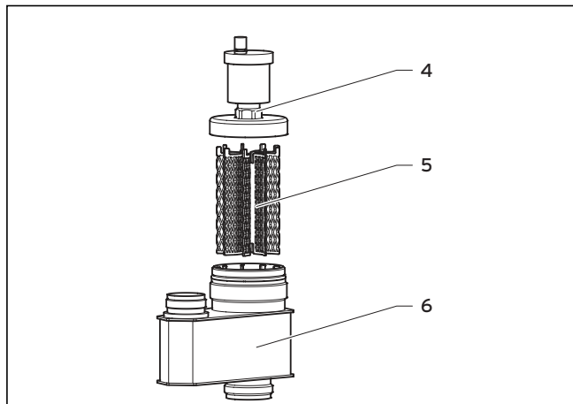
Рис. 8.9 Очистка фильтра
