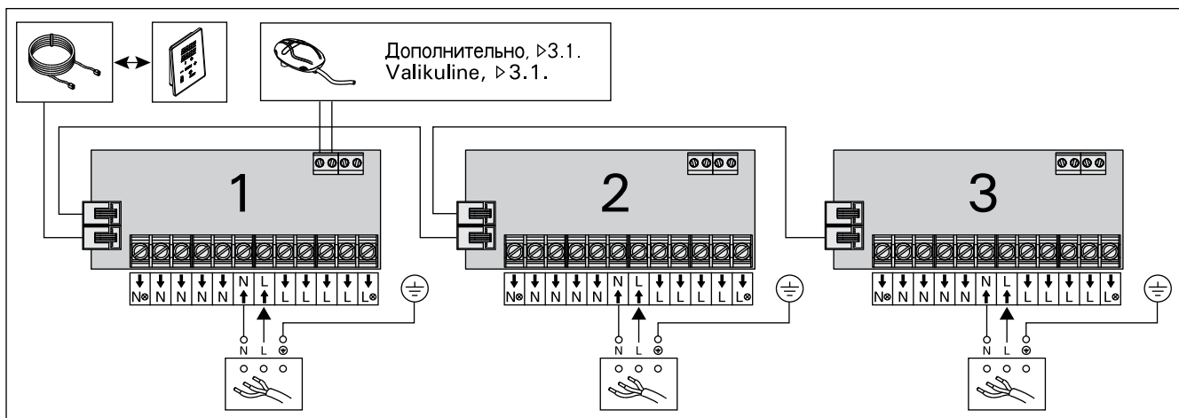
Рисунок 8. Multidrive
