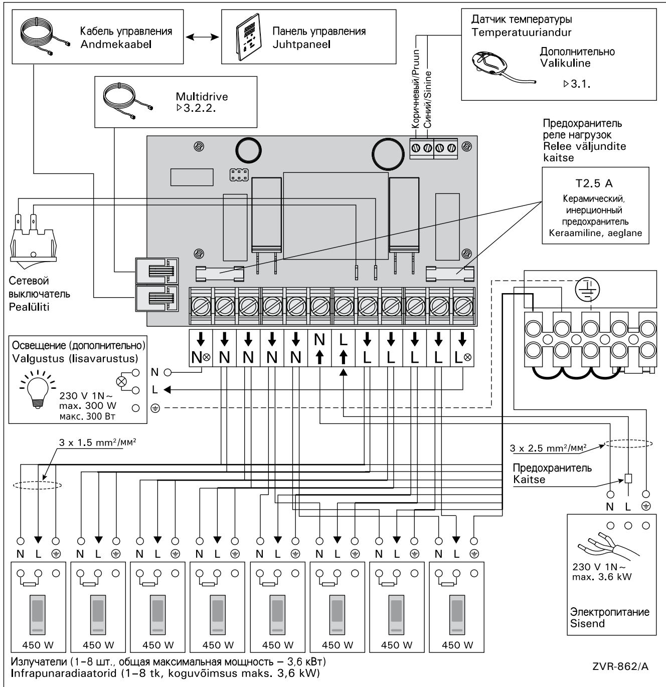
Рисунок 7. Электрические подключения
