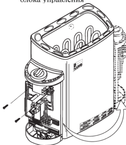
Fig. 3B Рис. 3Б Remise de l'unité de commande incorporée Перемещение встроенного блока управления
