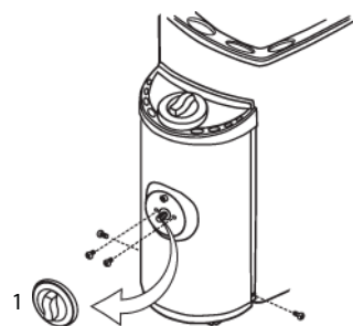
Fig. 4 Рис. 4 Connexion des câbles Соединение кабелей
