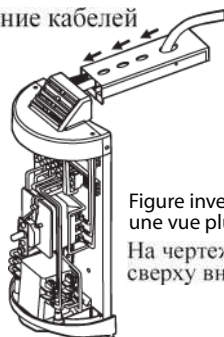
Fig. 4 Рис. 4 Connexion des câbles Соединение кабелей
