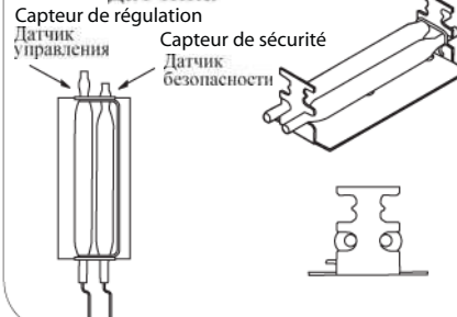
Рис. 8 | Местонахождение датчика
