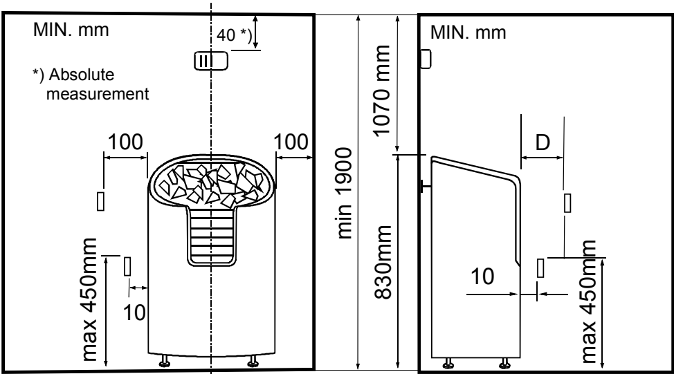
Рисунок 4 Безопасные расстояния
