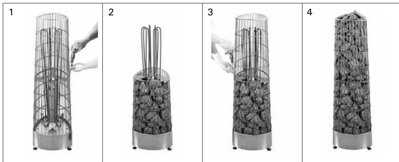
Рисунок 1. Укладка камней
