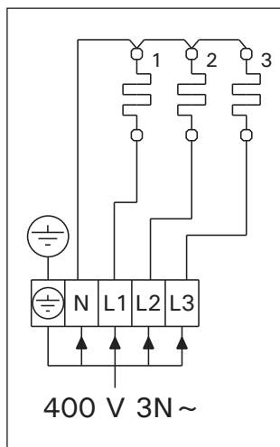
Рисунок 15. Электромонтаж каменки M-E Joonis 15. M-E-kerise elektriühendused
