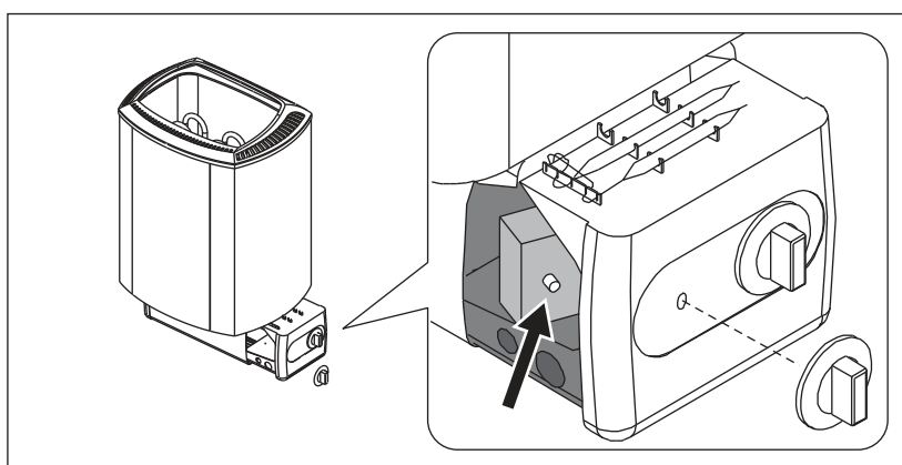
Рисунок 11. Кнопка сброса защиты от перегрева
