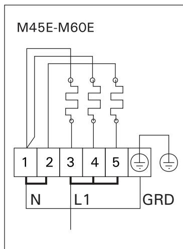
Рисунок 14. Электромонтаж каменки M-E (подключение в 1- фазной сети) Joonis 14. M-E-kerise 1-faasilised elektriühendused
