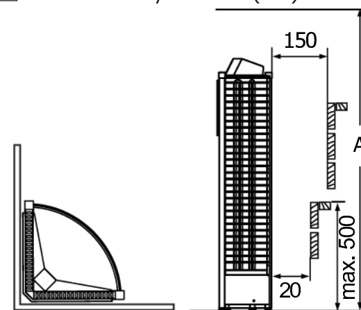
Рис. 2 Fig. 2 Минимальные безопасные расстояния, мм Minimum Safety Distances (mm)
