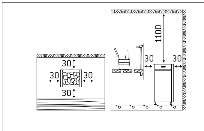
Рисунок 5. Расстояния безопасности (все размеры приведены в миллиметрах) Joonis 5. Kerise miinimum ohutuskauused (kõik mõõtmised millimeetrites)
