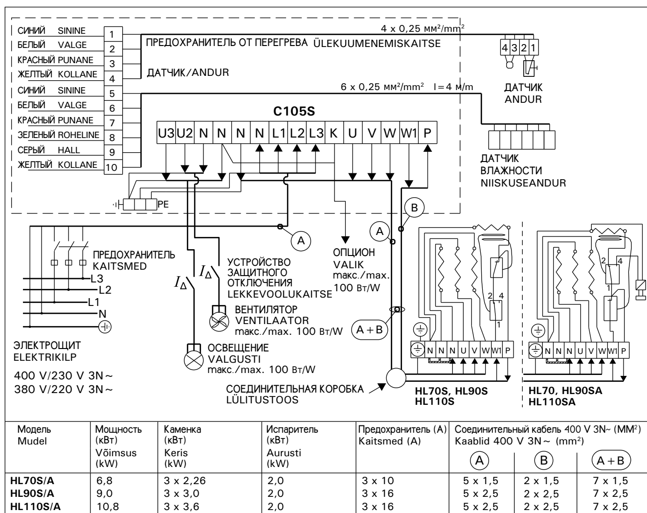
Рисунок 13. Электромонтаж пульта управления C105S и каменки HLS(A) Joonis 13. Juhtimiskeskuse C105S ja HLS(A)-kerise
