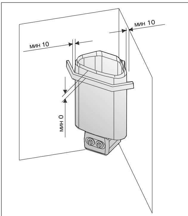
Рисунок 8. Защитное ограждение
