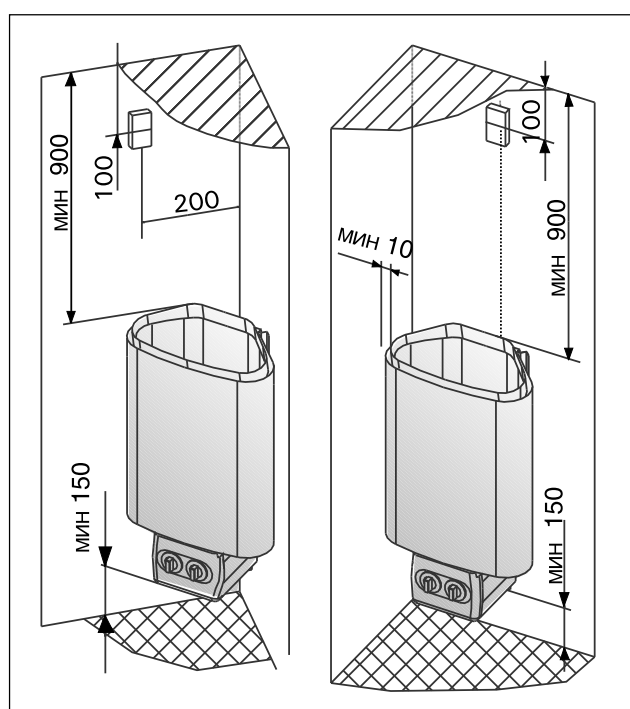
Рисунок 14. Установка датчика
