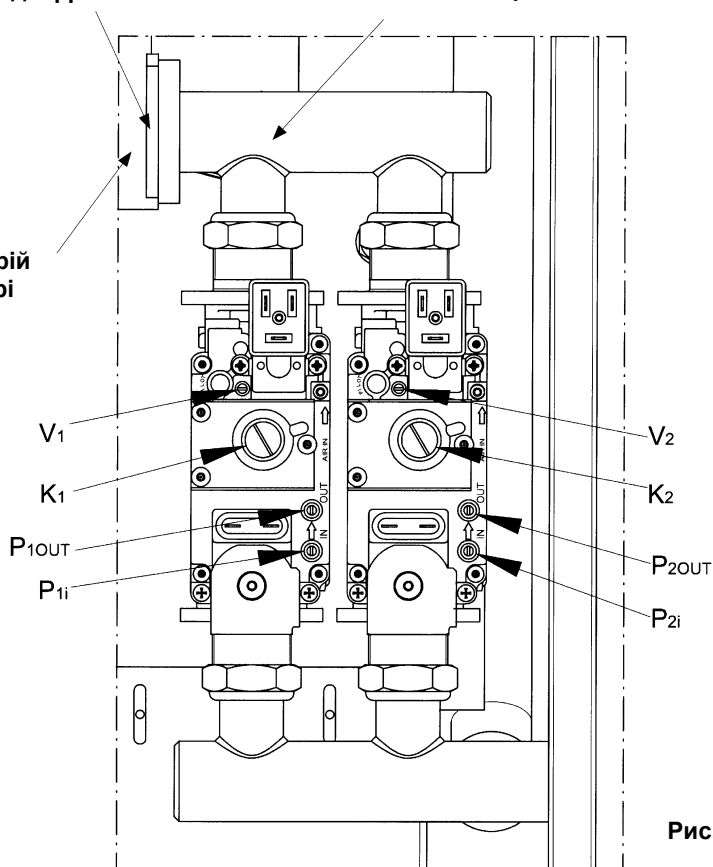
Клапанный коллектор
