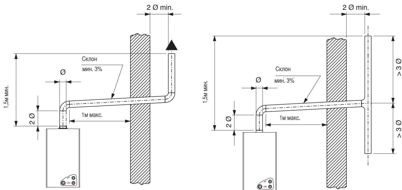
Рис. 9 – Подсоединение к дымоходу модели CTN
