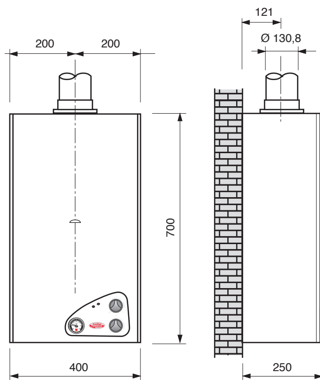
Рис.10 – Габаритные и разметочные размеры для подключения к дымоходу модели CTN
