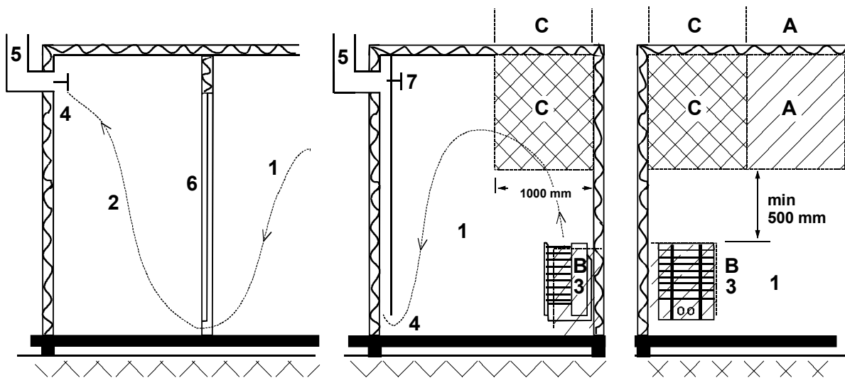
Рисунок 1. Вентиляция сауны
