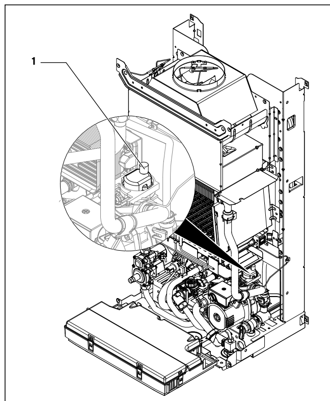
Рис. 6.1 Быстродействующий воздухоотводчик
