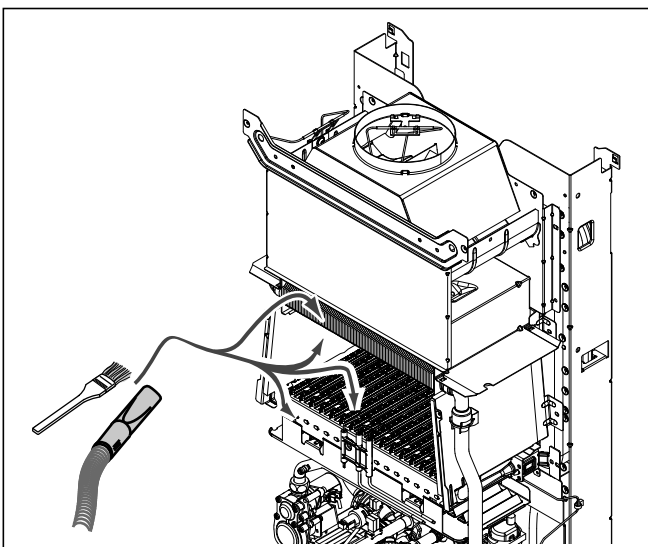
Мал. 8.1 Очищення палика і первинного теплообмінника без демонтажу деталей (незначне забруднення)
