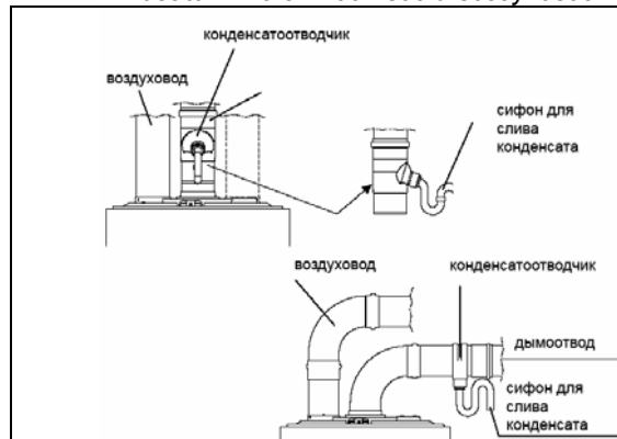
Раздельные дымоотвод и воздуховод
