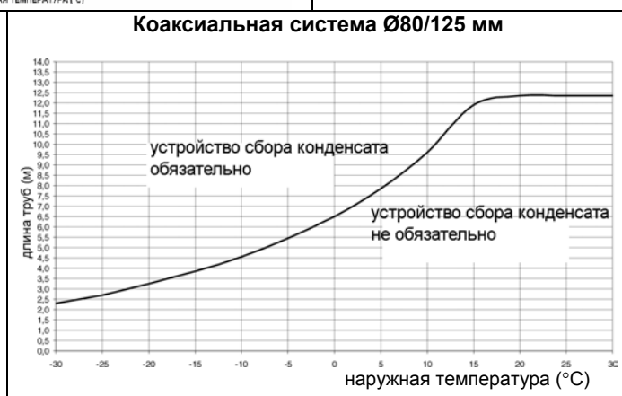
Коаксиальные дымоотвод/воздуховод
