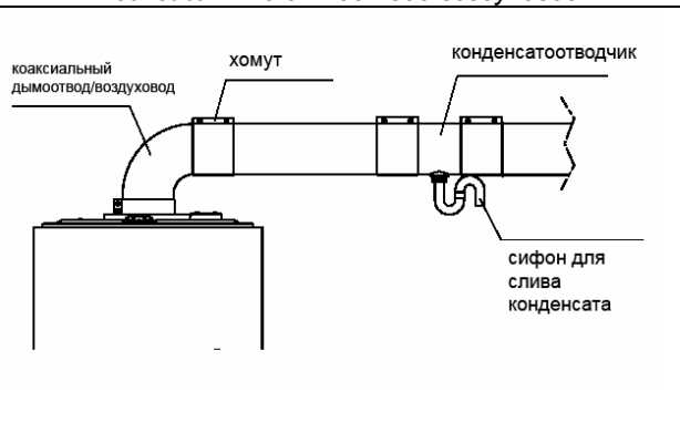
Коаксиальные дымоотвод/воздуховод
