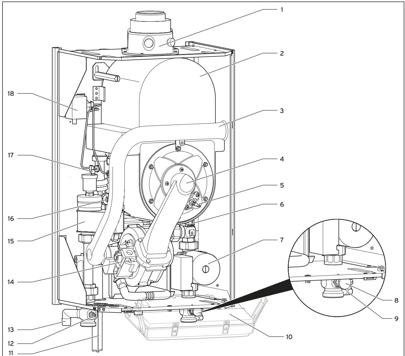
Рис. 2.1 Функциональные элементы
