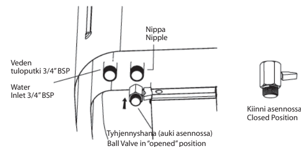
Kuva 1 Veden tuloputken kiinnitys (liitin sisältyy) Fig. 1 Connection pipe (hose included)
