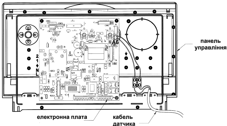
Рис. 8: Приєднання датчика вуличної температури
