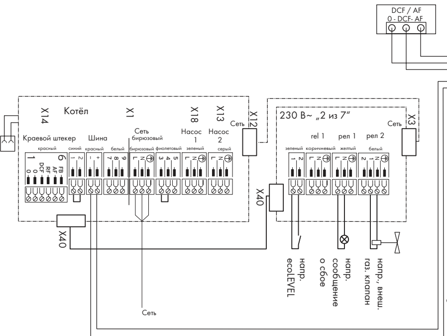
Рис. 5.15 Подключение регулятора VRS 620 или VRS 630
